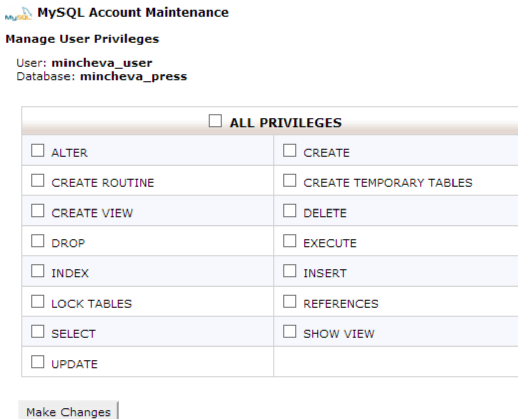
Фиг.3. Задаване на привилегии на mysql потребителя
